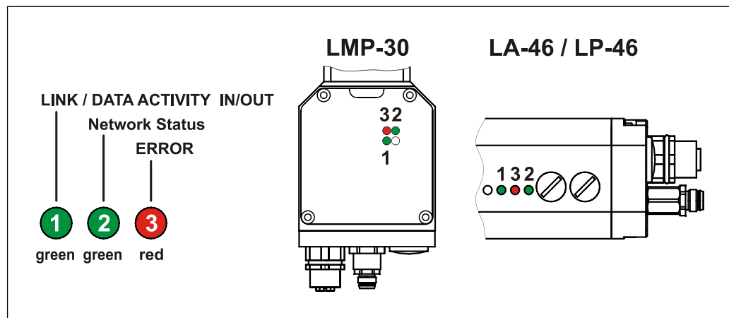
Abbildung 4: EtherNet/IP™ Diagnose-LEDs
